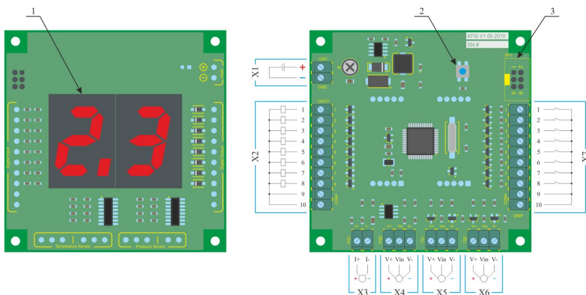
Рисунок 13. Блок управления
