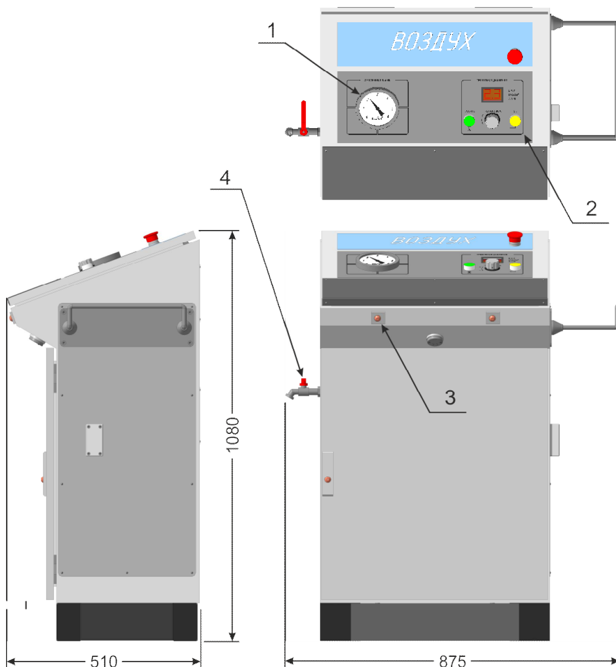
Рисунок 3. Пневмоавтомат, внешний вид
