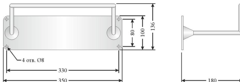
Рисунок 16. Кронштейн выходного рукава
