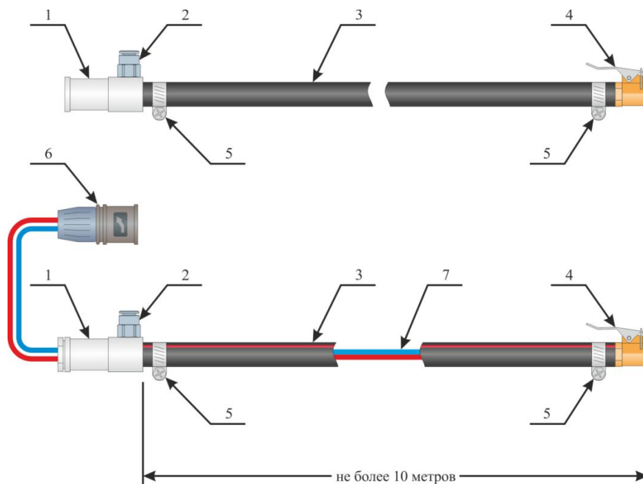
Рисунок 14. Выходной рукав: летний (вверху) и зимний (внизу)
