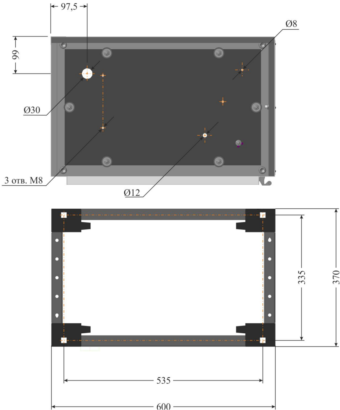
Рисунок 9 Расположение монтажных отверстий для крепления компрессора и пневмоавтомата
