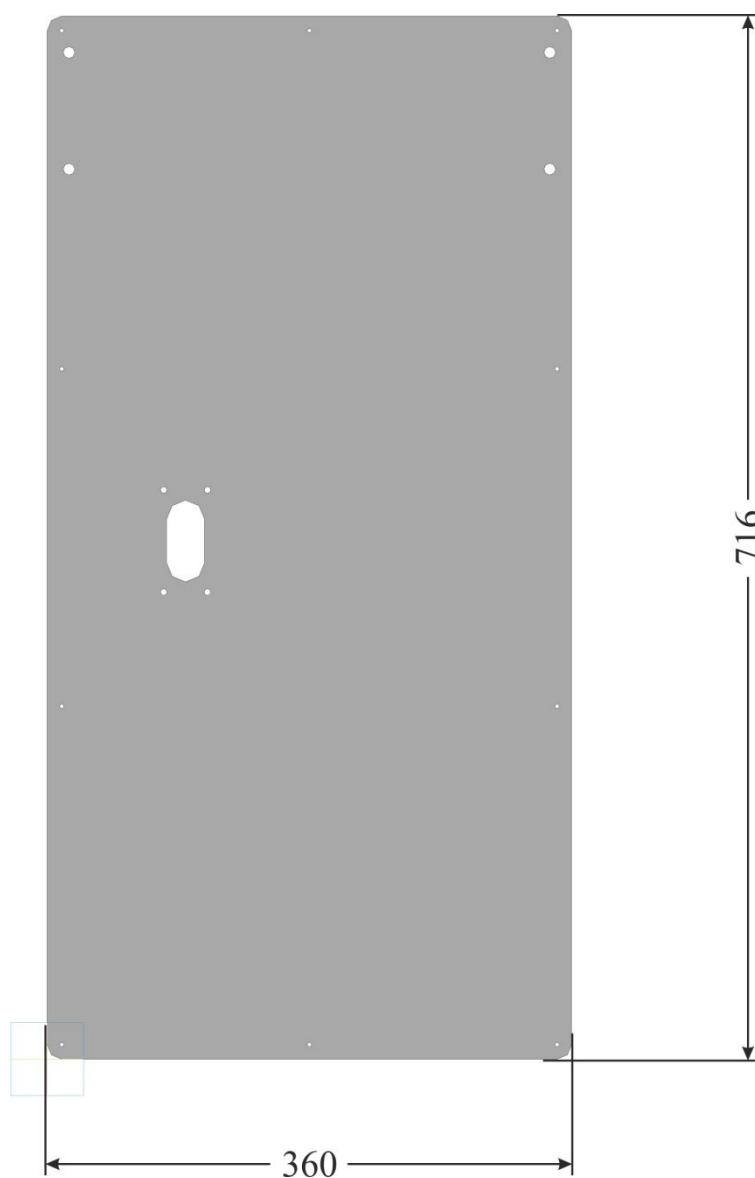
Рисунок 15. Защитный лист
