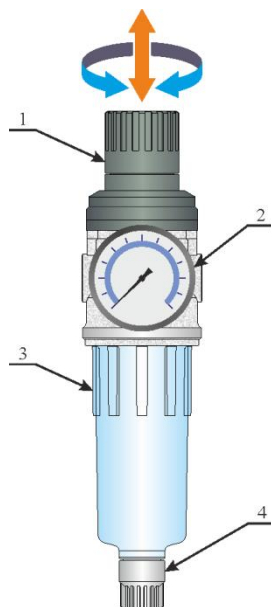
Рисунок 10. Блок подготовки воздуха
