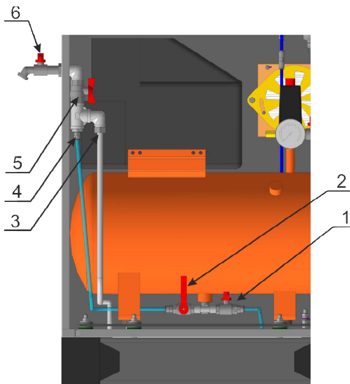
Рисунок 7 Пневмоавтомат с краном долива воды
