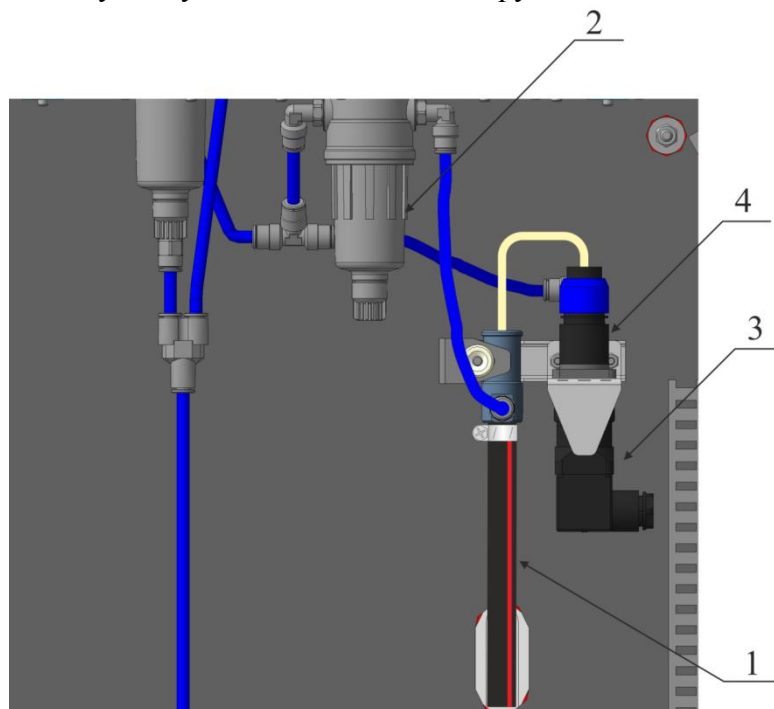
Рисунок 8 Пневмоавтомат, компоновка в зоне крепления выходного рукава
