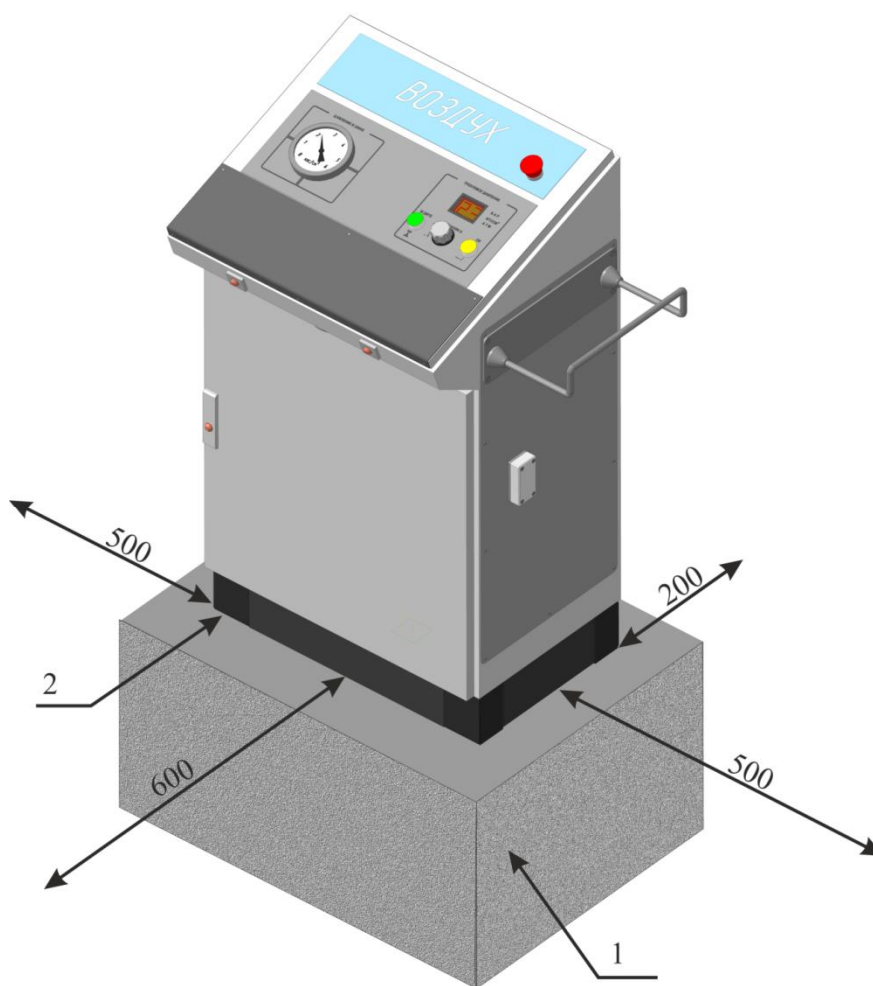
Рисунок 18. Рекомендуемая схема расположения пневмоавтомата
